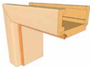
Řez obložkovou zárubní síla zdi od 5 cm, límce 6 cm
